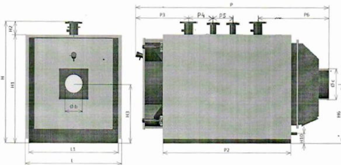
Мал 3. Зовнішній вигляд котлів SAB 0.95-1,15.
