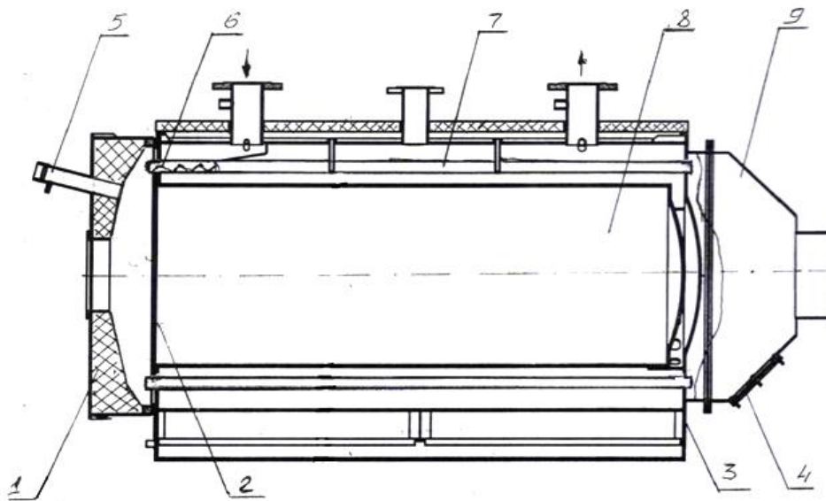
Малюнок 1- Будова котла.
