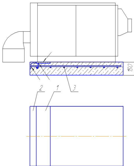
Малюнок 6 - Схема встановлення котла. 1-сталева закладна; 2-кутник; 3-арматура
